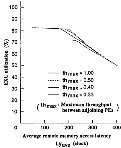
図 5: ネットワーク性能による演算部稼働率の変化 (Matrix)
