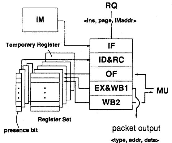
図 2: Function Unit 構成図
