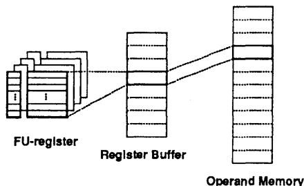
図 7: Datarol-II プロセッサのメモリ階層
