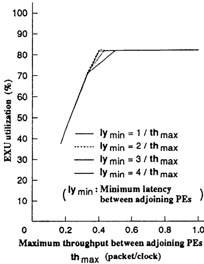
図 5: ネットワーク性能による演算部稼働率の変化 (Matrix)
