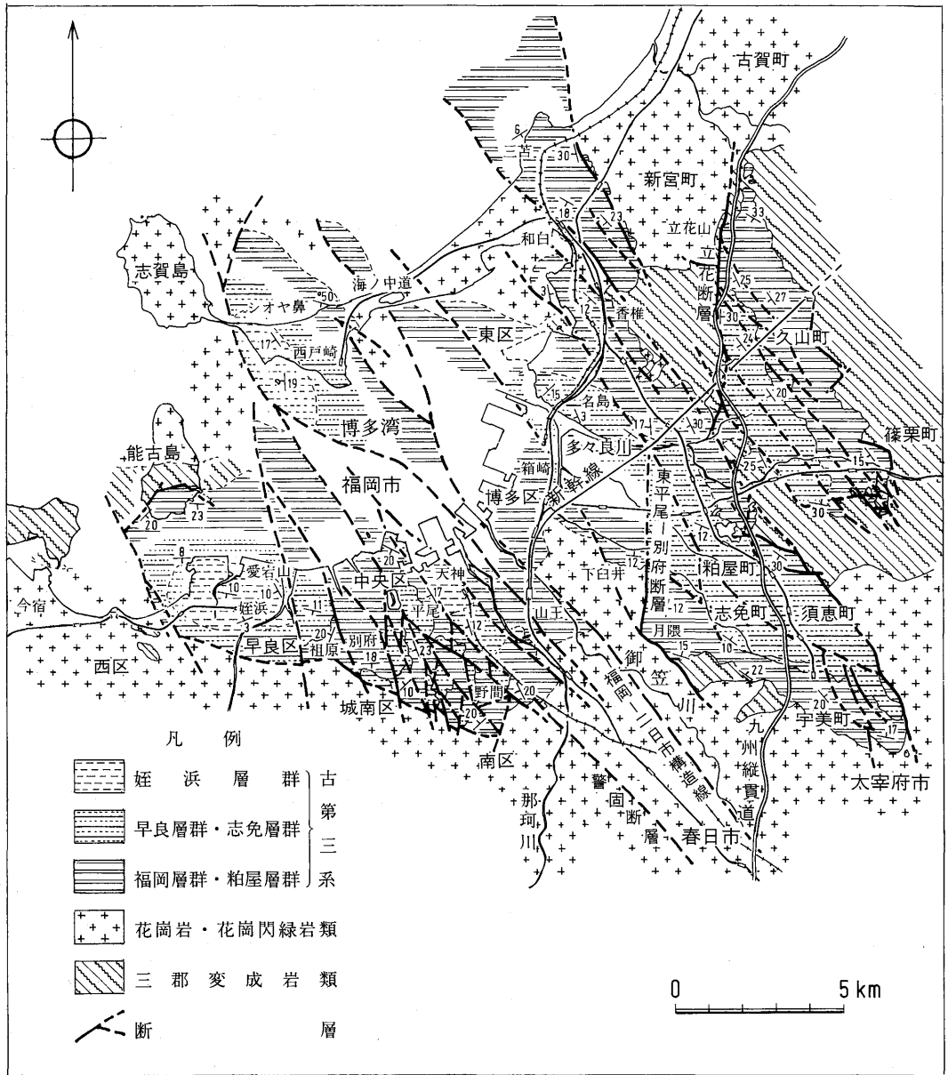
第8図 福岡-粕屋炭田地質図
