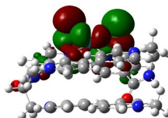
MO193 (HOMO-1)
