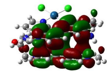
MO194 \alpha (HOMO)
