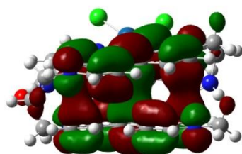
MO194 (HOMO)
