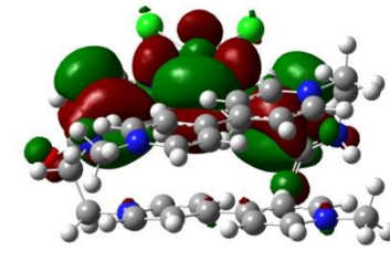
MO195 \alpha (LUMO)
