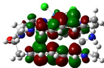
MO203 (LUMO+8)
