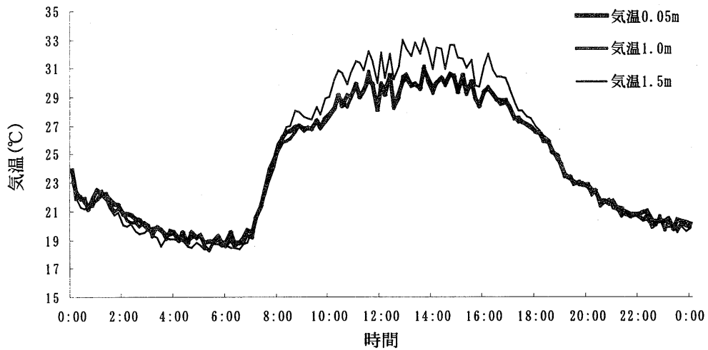
図9 気温
