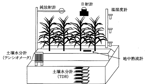
図6 気象観測装置の設置状況
