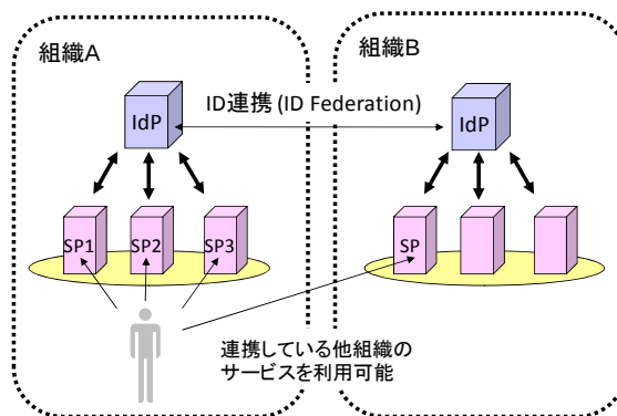
図 2 組織間での ID 連携
