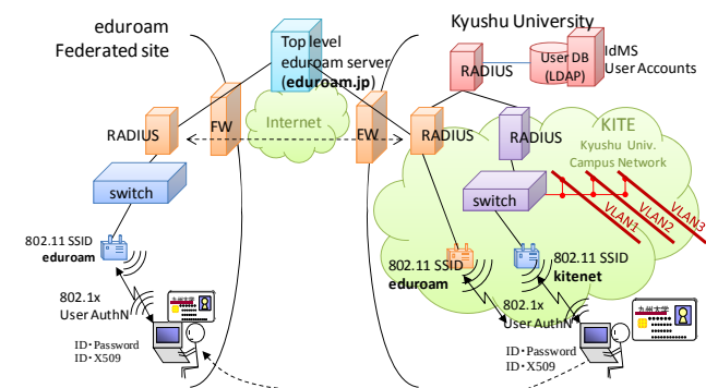
図 5 九州大学の eduroam 環境
